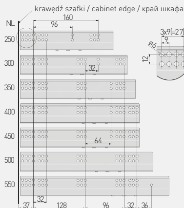
Rozstaw otworów montażowych Mounting dimensions Монтажные отверстия
