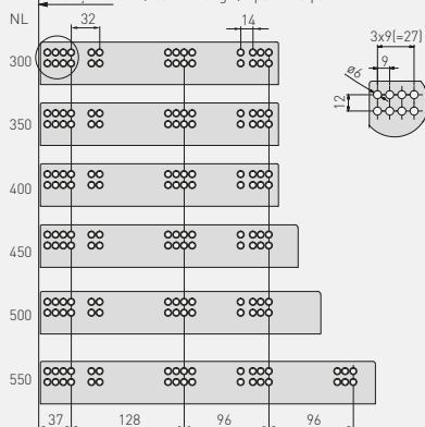
Rozstaw otworów montażowych Mounting dimensions Монтажные отверстия
